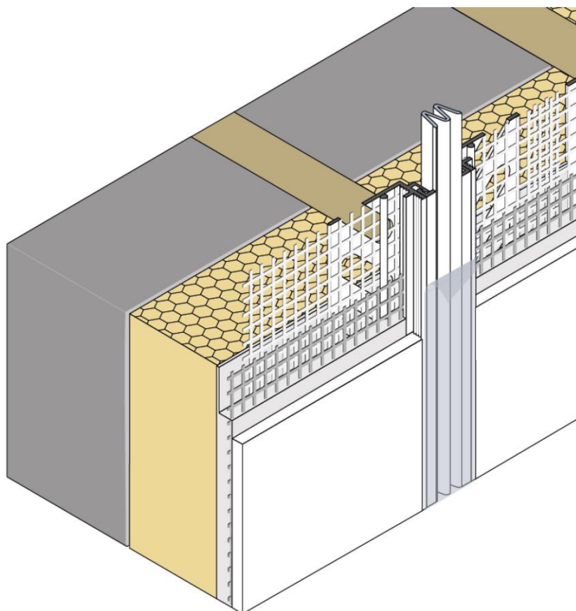
obr. 2: StoProfile Move V 2 – zabudovanie na ploche
