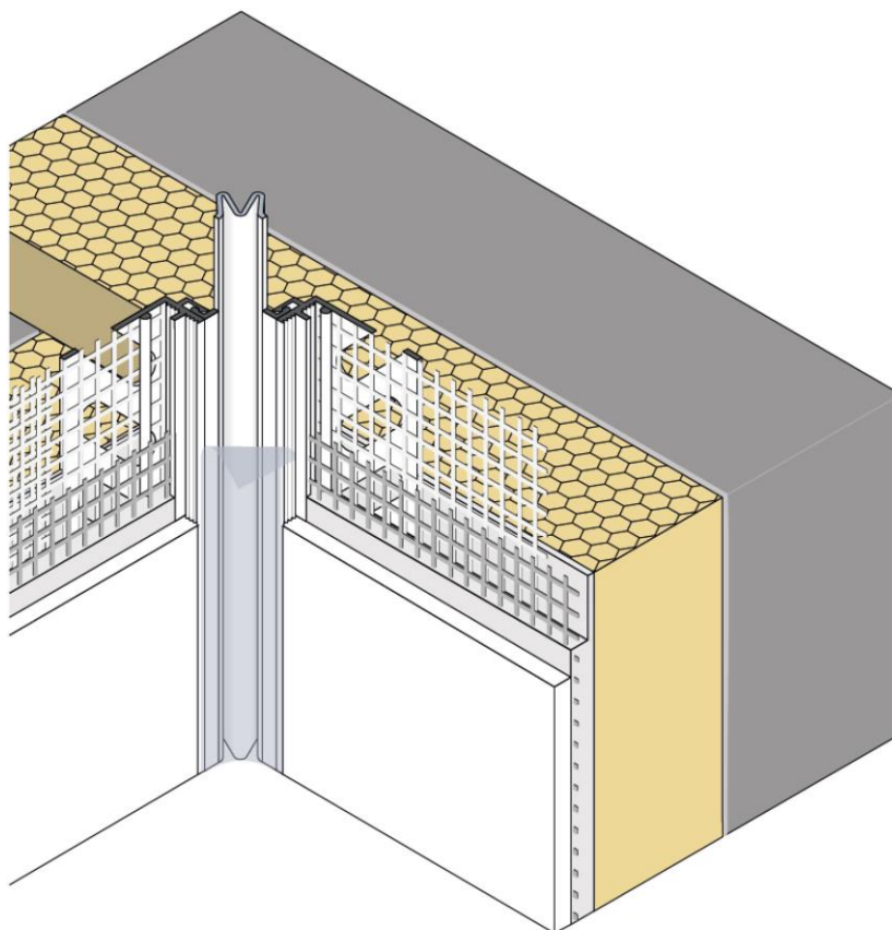
obr. 3: StoProfile Move V 2 – zabudovanie vo vnútornom rohu
