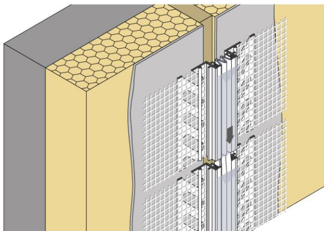
obr. 4: StoProfile Move V 2 – vytvorenie vertikálneho styku
