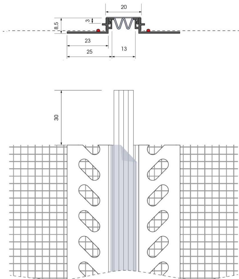
obr. 1: StoProfile Move V 2 – geometria profilu a rozmery
